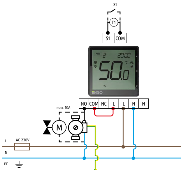
a) Siurblio ir (arba) pavaros prijungimo schema
