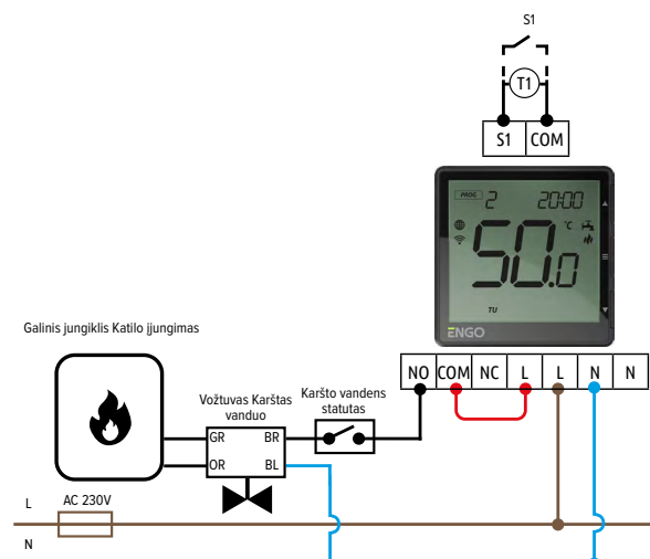
b) Karšto vandens vožtuvo prijungimo schema per karšto vandens statinį.
