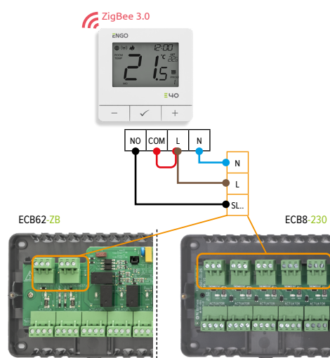
c) Prijungimo prie valdymo bloko schema
