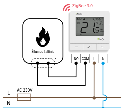
a) Prijungimo prie šilumos šaltinio schema
