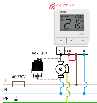
b) Siurblio ir (arba) pavarų siurblio prijungimo schema
